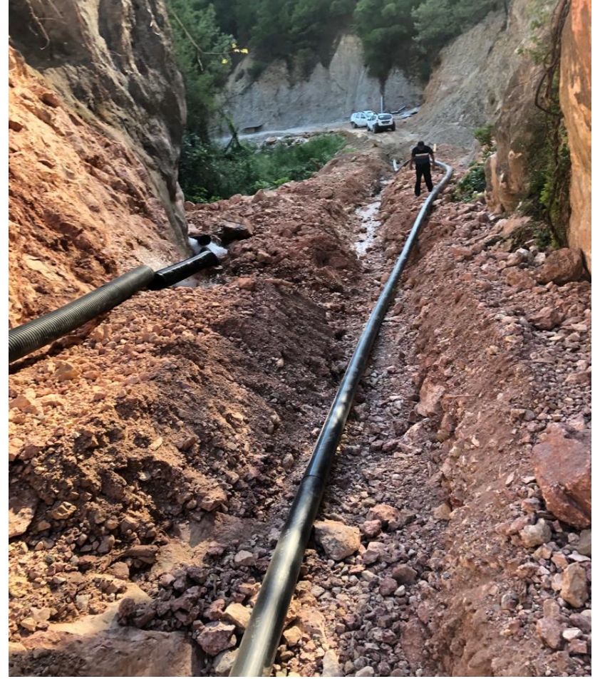
Söğüt Akçasu-Yakacık Cazibeli İsale Hattı
